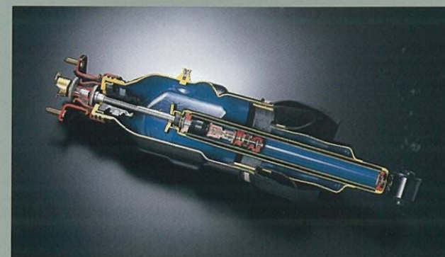
電子制御エアサスペンション
