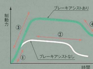
ブレーキアシストの考え方
